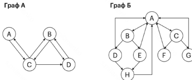
Рис. 1: Примеры графов
